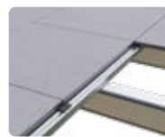
Structure pour habillage «Grés» pour dalles de 60cm x 60cm x 2cm (dalles non fournies)
